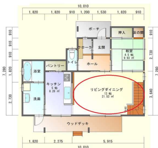
1 階
